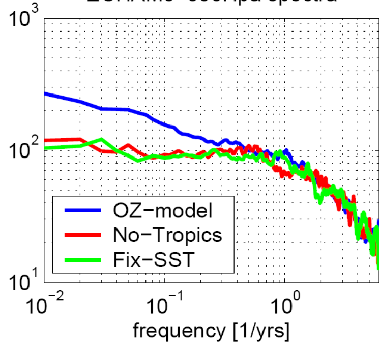
b) ECHAM5 500hPa spectra
